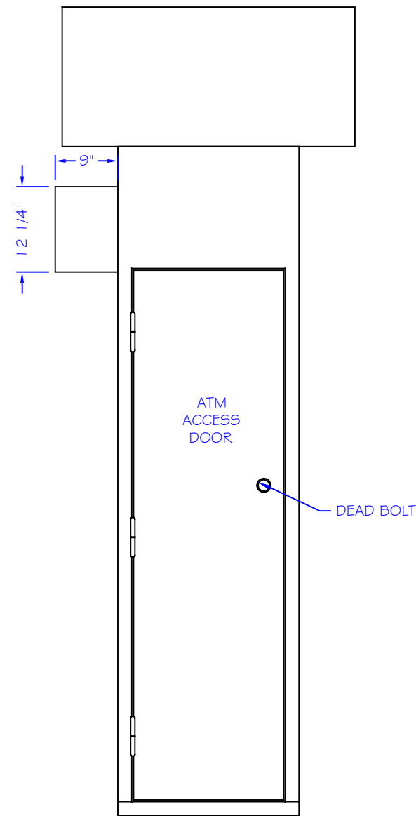
REAR ELEVATION SCALE: 1/2" = 1'
