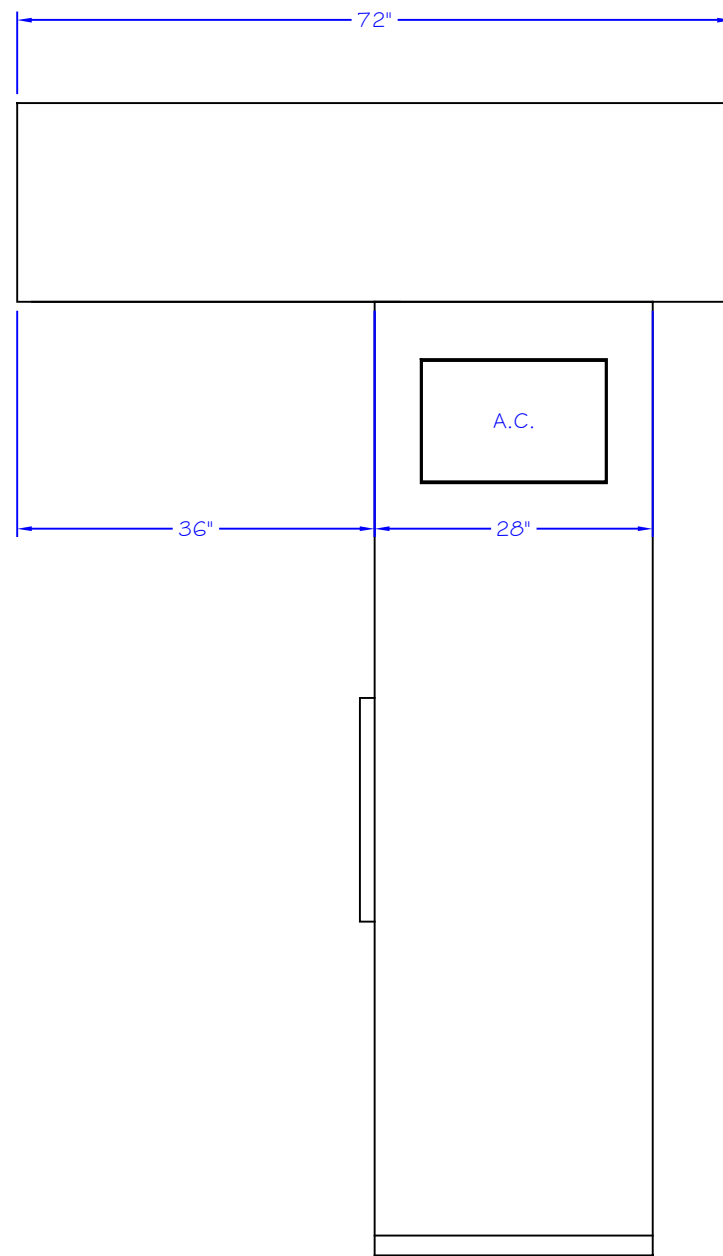
RIGHT ELEVATION SCALE: 1/2" = 1'
